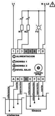
K1, K2 = arrancadores F3 = foco piloto
